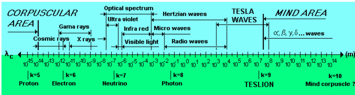
Slika 2, EM spektar u Modelu KGE
